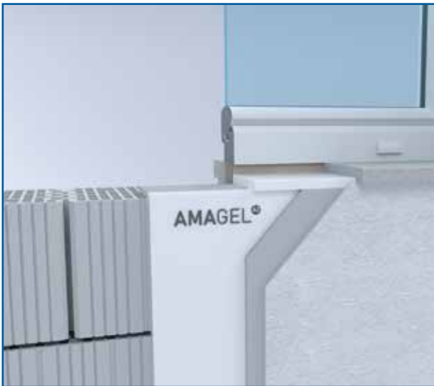
PONTS THERMIQUES
