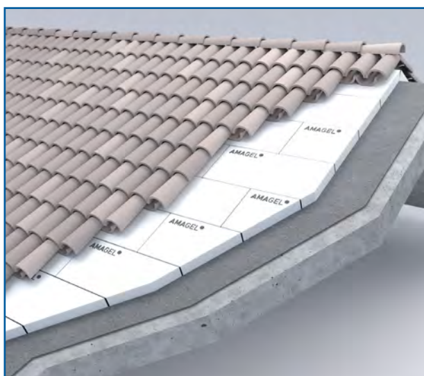
TECHOS
