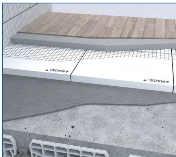
FORJADOS ENTREPLANTA
